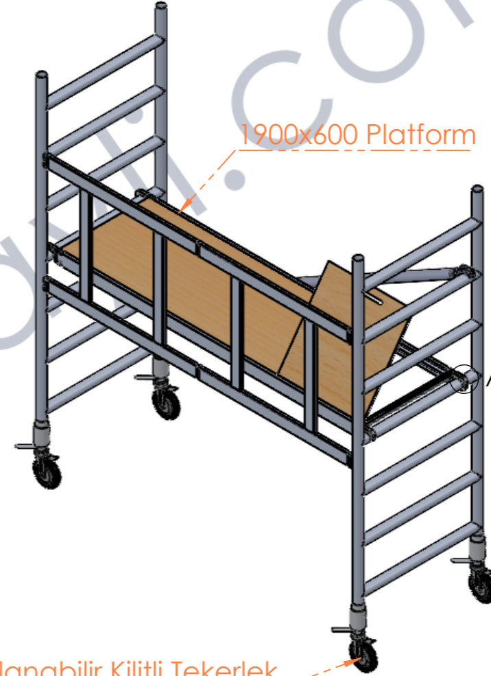
Ayarlanabilir Kilitli Tekerlek
