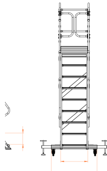
מבט חזית
