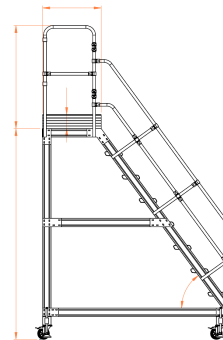
מבט צד
