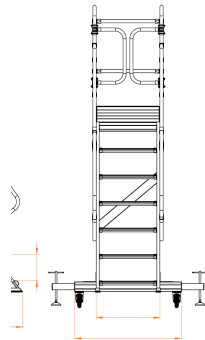
מבט חזית
