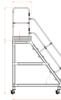
מבט צד
