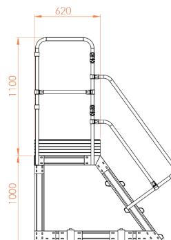
מבט צד
