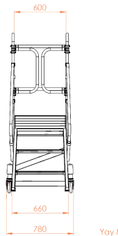
מבט חזית
