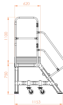
מבט צד
