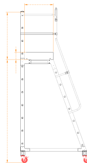
מבט צד גובה פלטפורמה 217 ס"מ
