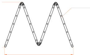
תצורת פיגום גובה 141.4 ס"מ
