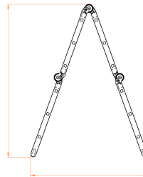
תצורת A גובה 169.1 ס"מ
